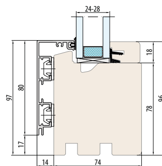
SYSTÈME ESPERIA LIFE 74 ALU-Fix
