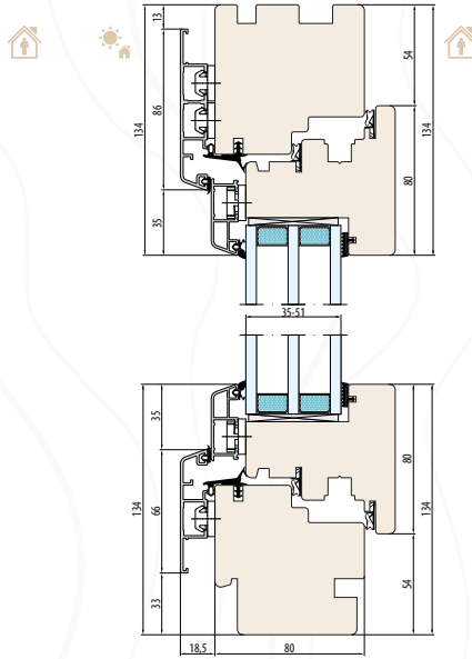
SYSTEME NATURO 80 ALU GEMINI CLASSIC découpe pour l'appui de fenêtre intérieur et extérieur
