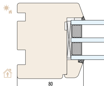
SYSTÈME NATURO 92 -Fix SECTION HORIZONTALE B-B
