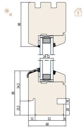
SYSTÈME NATURO 68-Fix découpe pour l'appui de fenêtre intérieur et extérieur
