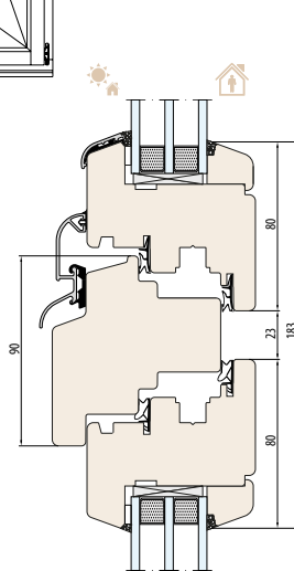
SYSTÈME NATURO 80 traverse 90 mm
