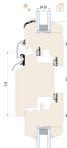
SYSTÈME NATURO 68 traverse 115 mm
