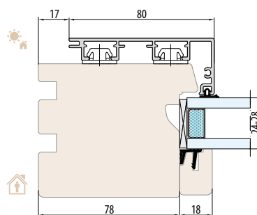
SYSTÈME ESPERIA LIFE 74 ALU-Fix SECTION HORIZONTALE B-B
