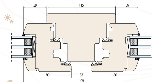
SYSTÈME NATURO 80 meneau fixe 115 mm (section horizontale)
