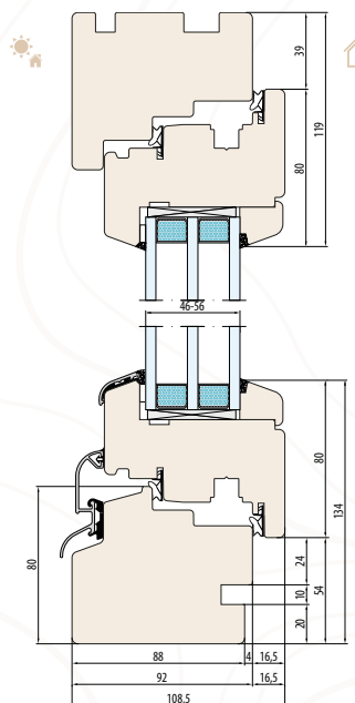
SYSTÈME NATURO 92 découpe pour l'appui de fenêtre intérieur
