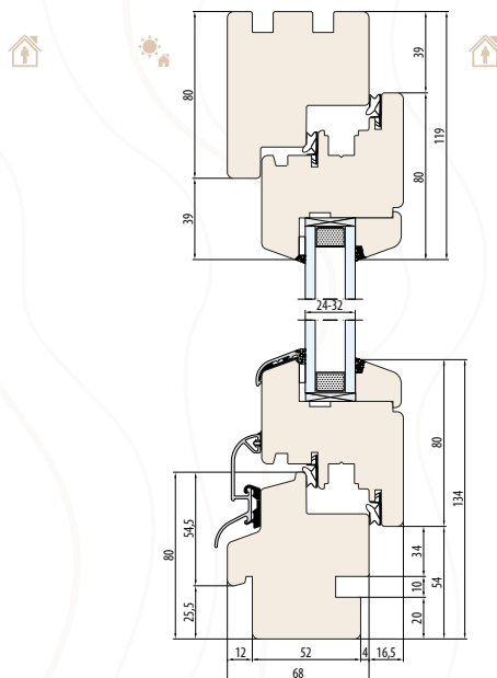
SYSTÈME NATURO 68 découpe pour l'appui de fenêtre intérieur et extérieur
