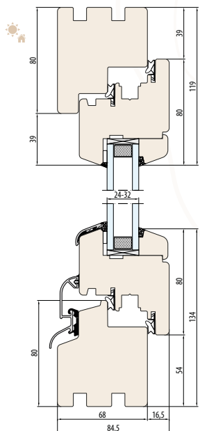
SYSTÈME NATURO 68 sans découpe pour l'appui de fenêtre
