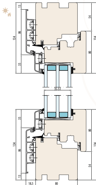
SYSTEME NATURO 80 ALU GEMINI CLASSIC sans découpe pour l'appui de fenêtre
