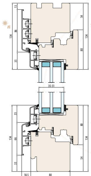
SYSTEME NATURO 80 ALU GEMINI CLASSIC découpe pour l'appui de fenêtre extérieur
