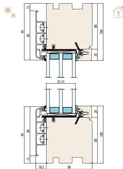
SYSTÈME NATURO 80 ALU-Fix
