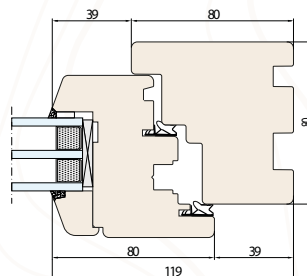
SYSTÈME NATURO 80 découpe pour l'appui de fenêtre intérieur
