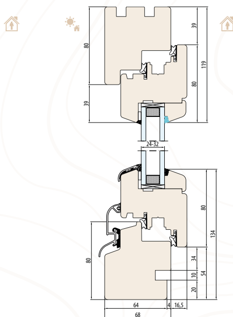
SYSTÈME NATURO 68 découpe pour l'appui de fenêtre intérieur
