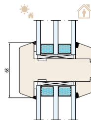
SYSTÈME NATURO 92 meneau structurel 68 mm
