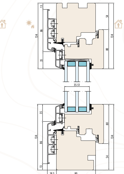
SYSTEME NATURO 80 ALU GEMINI CLASSIC découpe pour l'appui de fenêtre intérieur
