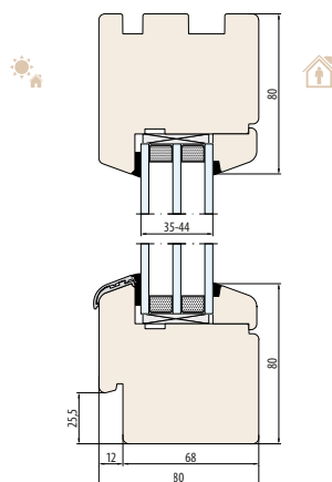
SYSTÈME NATURO 80-Fix découpe pour l'appui de fenêtre extérieur
