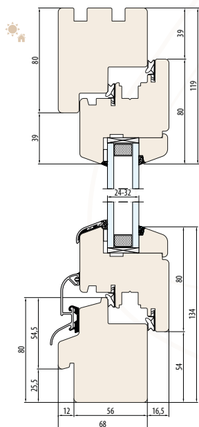
SYSTÈME NATURO 68 découpe pour l'appui de fenêtre extérieur
