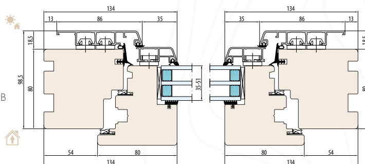
SYSTEME NATURO 80 ALU GEMINI CLASSIC découpe pour l'appui de fenêtre extérieur
