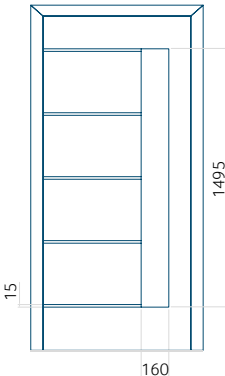
Dessin technique
